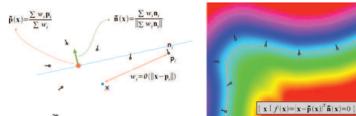
Modélisation 3D
